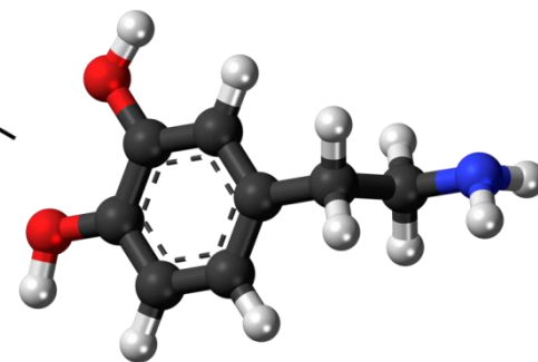
dopamina
