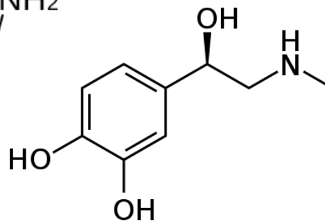
adrenalina
