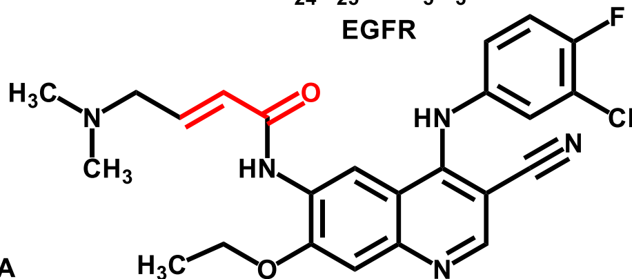
Pelitinibe
