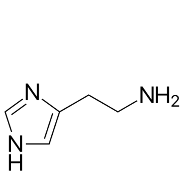
histamina
