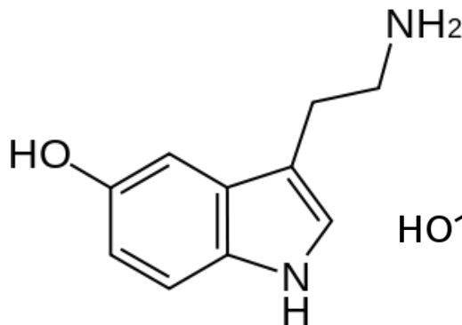
serotonina
