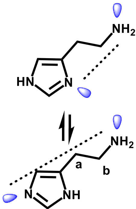
histamina
