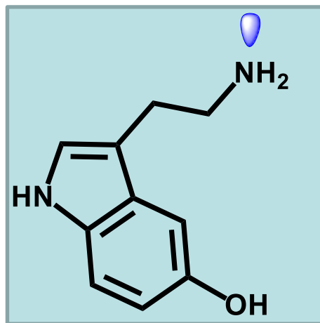
serotonina
